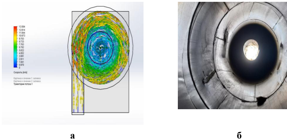
Рис. 1. Вид сверху на внутреннюю часть циклона пылеуловителя новой конструкции и траектория вращения пылевых частиц.
