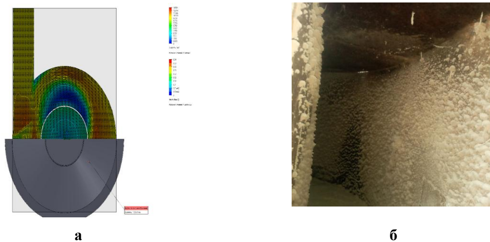
Рис. 2 Внутренний вид на входной патрубок циклона пылеуловителя новой конструкции и вид на входной поток пылевых частиц
